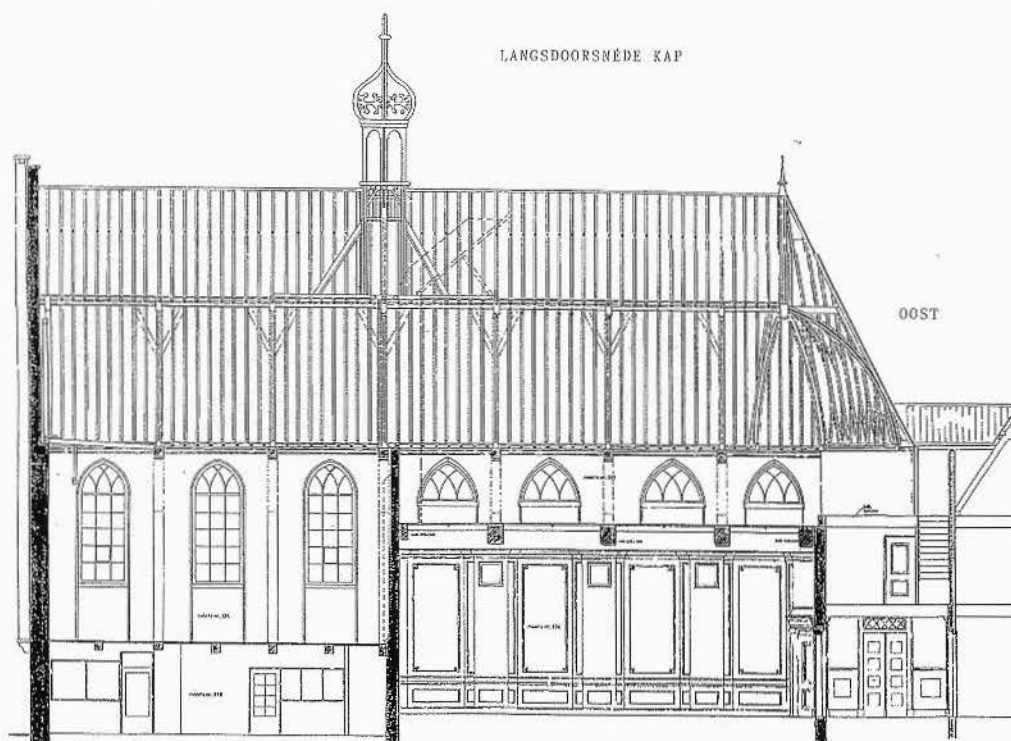
Afbeelding 1 geeft een langsdoorsnede van het kerkje aan de tuinzijde te zien, met de verbouwingen in de zijgevel die in de loop der tijd hebben plaatsgevonden.
